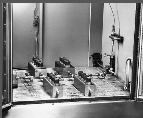
Impulse Test
